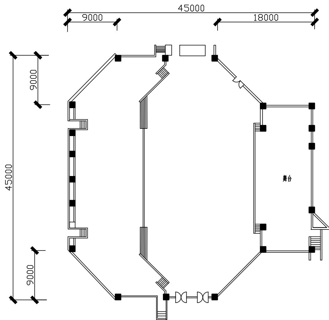
1#会议厅平面
